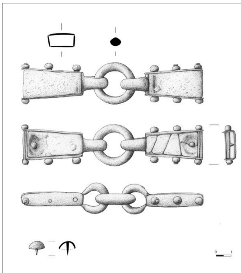
Fig. 3. Dibujo de las piezas. (Autora: Patricia Fuentes Melgar).
